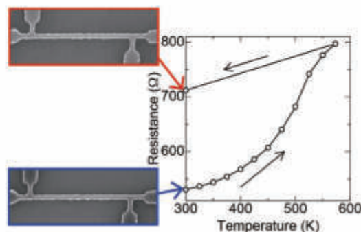
銅-ニッケル二層細線の熱履歴メモリ (リフトオフプロセス使用)
