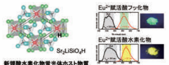
新規酸水素化物蛍光体ホスト物質
