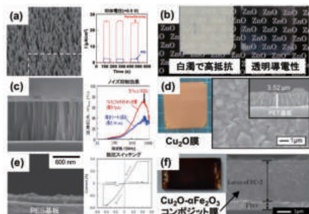
(図1) (a) ナノロッドアレイ型光電極、(b) 透明導電 \text{ZnO} 膜、(c) 電磁ノイズ抑制フェライト膜、(d) 半導体 \text{Cu}_2\text{O} 膜、(e) 抵抗変化型メモリ用 \text{CeO}_2 膜、(f) スーパーキャパシタアノード用 \text{Cu}_2\text{O}-\alpha\text{Fe}_2\text{O}_3 膜
