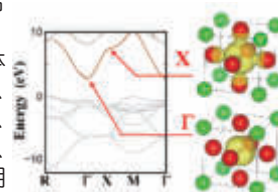
図3 量子計算で描いた SrGeO 3 の波動関数。
