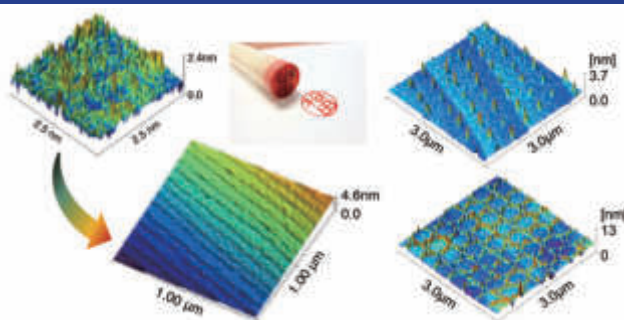
フレキシブル基板表面での原子ステップ（左）、1nmドット配列（中）、1nmメッシュ（右）形成
