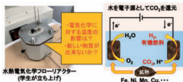
図3（左）学生が立ち上げた水熱電気化学フローリアクター （右）鉱物を触媒として使い、CO 2 を有用物質へと変換
