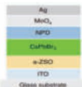
図2. アモルファス \text{Zn-Si-O} (ZSO) の新たな電荷輸送層を用いるペロブスカイト EL の素子構造および発光写真。右図はプラスチック基板上に作製されたペロブスカイト EL。
