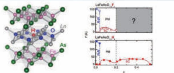
鉄系超伝導体 \text{LaFeAsO}_{1-x}\text{H}_x \text{O}^{2-} を水素アニオン \text{H}^{-} に置換することで高濃度電子ドーピングを実現(Nat. Commun. 3, 943)
