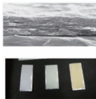
図3 硫酸浴中で作製したアルミナ皮膜の断面SEM像（上）、シュウ酸浴中で作製したアルミナ皮膜の外観（下）
