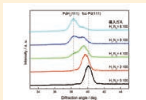
図6 X線回折法によるPd/AlN極薄膜の水素化その場観察
