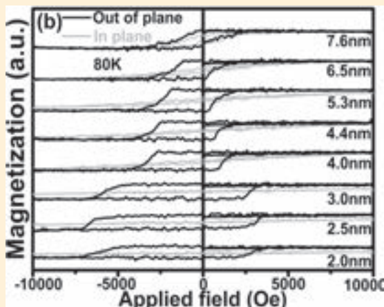
図5は CoPt/CoO ナノヘテロ多層膜の磁化曲線です。
