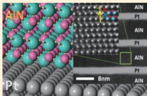
図2 AlN/Pt多層膜の原子分解能電子顕微鏡とAlNの成長様式
