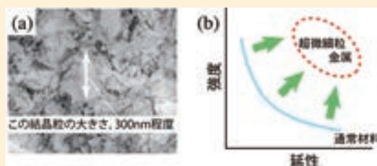
図2 (a)はNi多結晶中の超微細結晶粒を示す透過型電子顕微鏡写真である。超微細粒金属は、(b)の赤点線の領域のような強度と延性の両方に優れた材料になると期待されている。
