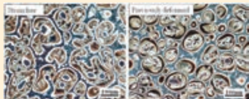
図4 Weck's 試液で腐食することによって現れた、球状化した固相内の溶質偏析と初晶デンドライトの形態変化 (AC4CH 合金の半熔融材：青い部分は急冷された残留液相)
