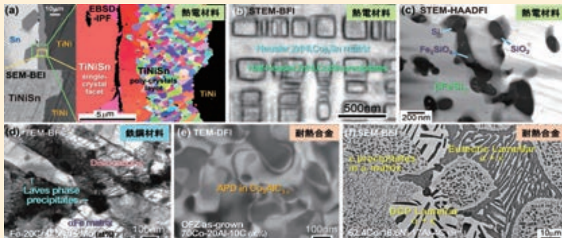
図 (a) \text{TiNi}/\text{Sn} 固液界面での Half-Heusler \text{TiNiSn} 多結晶層と単結晶 facet の形成, (b) Heusler \text{Zr}(\text{Ni},\text{Co})_2\text{Sn} 母相と Half-Heusler \text{Zr}(\text{Ni},\text{Co})\text{Sn} 析出, (c) 共析 \text{Si} と \text{Fe}_3\text{O}_4 の酸化還元焼結による \text{SiO}_2 分散 \beta\text{FeSi}_2 複相組織, (d) 強加工 \beta\text{Fe} 母相結晶粒界と粒内に析出する Laves 相 (\text{Fe},\text{Cr})_3(\text{Nb},\text{Mo}) , (e) \text{E}_{21} \text{Co}_3\text{Al} 単結晶の逆位相領域 APD, (f) 三形態共存の二相組織: \alpha\text{Co} 母相と \kappa\text{-Co}_3\text{Al} 析出, 共晶ラメラ, 不連続析出 DCP ラメラ。
