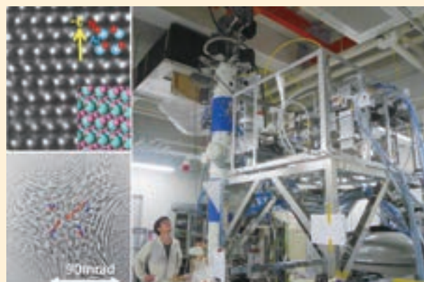
図3 左上：AINの超高分解能電子顕微鏡写真。左下：ロンチグラムの自動中心検出トレース。右：開発中の高周波加速TEMの外観
