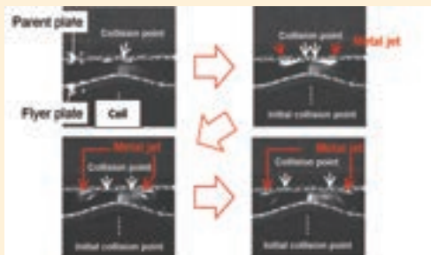
図1 高速ビデオカメラでとらえた電磁力衝撃圧接時の金属板の変形挙動と衝突点からのメタルジェット放出挙動 試験片：純Al板（厚さ1mm） 衝突時間：数マイクロ秒 推定衝突速度：500m/s
