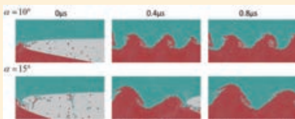
図2 Cu/Niの高速傾斜衝突界面におけるメタルジェット放出と波状界面形成（粒子法： \alpha は衝突角度、時間は衝突後の経過時間） ・衝突点から放出されたメタルジェットと衝突点前方の金属表面が干渉し、波状界面が形成 ・衝突角度の増加により波の波長と振幅が増加 ・ある衝突角度を超えると波が形成しなくなる
