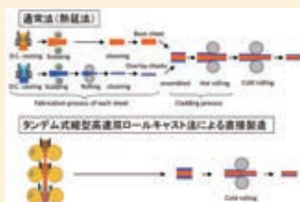
図3 本研究室で開発したタンデム式縦型高速双ロールキャスト法により、従来法に比べ大幅な省工程で、優れた特性を有するクラッドシートを製造することが可能である
