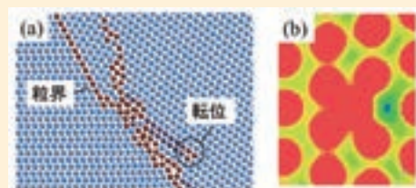
図3 計算科学によって転位の運動や阻害、結合の破断といったミクロな現象を捉えることができる。(a)は分子動力学計算で得られた粒界と転位が相互作用する様子、(b)は第一原理計算で得られた粒界近傍の電子密度を示す図である。
