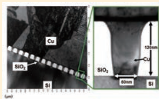
図 1. 半導体テストチップ (直径 60nm・深さ 200nm) へ超臨界ナノプレーティング (SNP) 法による埋込んだ Cu の TEM 像
