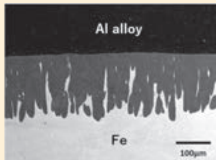
図2 鉄とAl合金を液相拡散接合法により形成された接合界面の組織。界面で生成している金属間化合物が固相の鉄に向かって成長するのが面白い
