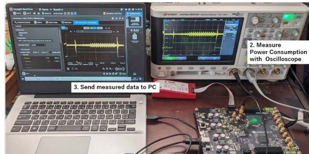
図4：電力波形を解析されても安全な組込みシステム
