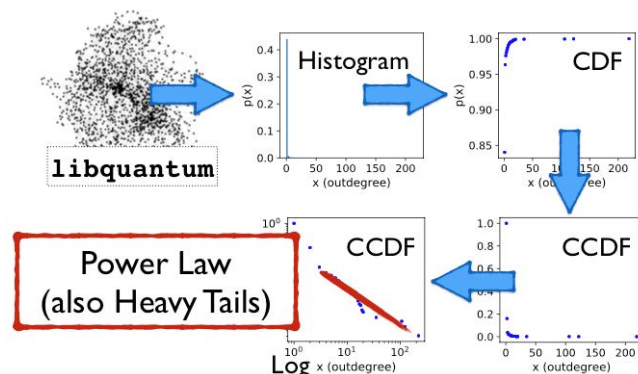
図 2：プログラムソーシャルネットワーク解析
