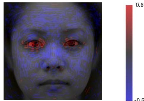
図3 新しい心理物理実験により顔認知に影響する部位やその効果を可視化する。
