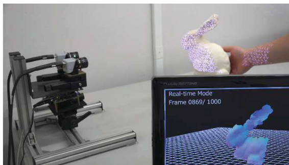
図 1 1000fps 形状センシング
