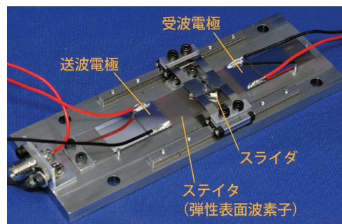
図1. 弾性表面波モータの原理と応用(上) 試作例(下:最大速度 1 \text{ m/s} , 最大推力 20 \text{ N} )
