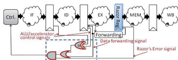
図 2：故障を検出・修正するアーキテクチャ
