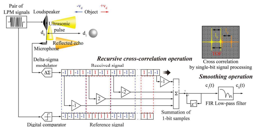
図2 エコーロケーションシステムと1bit 演算による相互相関信号処理
