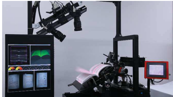
図 2 高速書籍電子化システム
