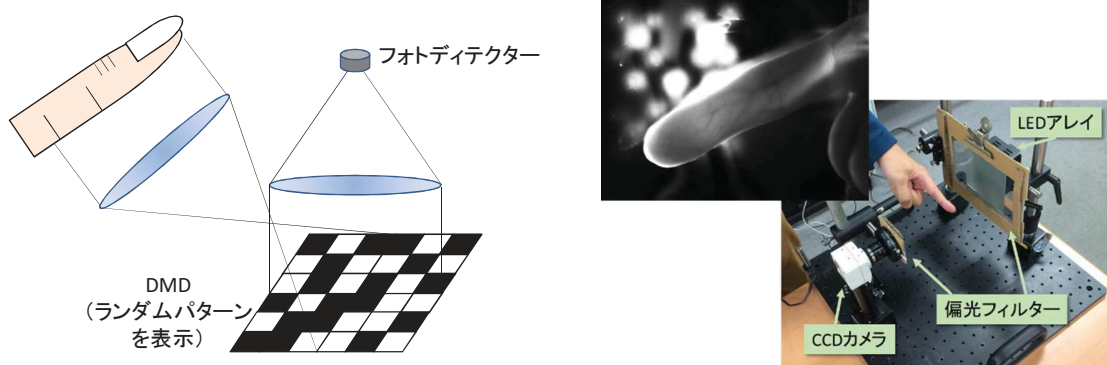
図 3. 圧縮センシングによる秘匿化生体画像の取得 図 4. 手振り型指静脈認証システム
