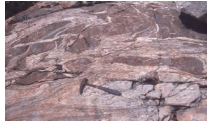
約 40 億年前の岩石
