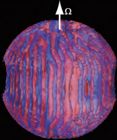
コア内部の渦分布のシミュレーション
