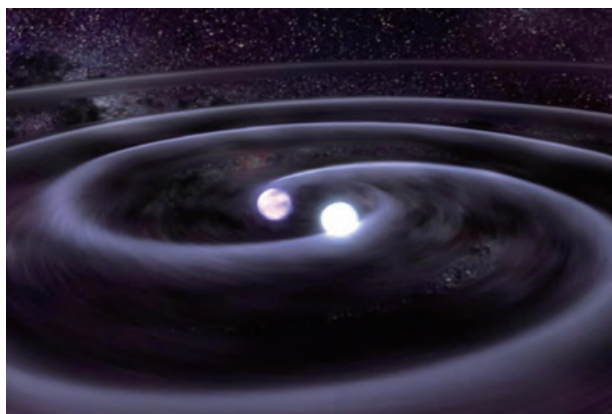
図 2. 中性子星合体の想像図。連星中性子星が重力波を放出することにより、軌道エネルギーと軌道角運動量を失い、徐々に軌道距離を縮めながら最終的に衝突する。©NASA
