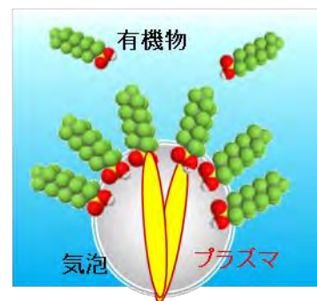
処理水中に多数のプラズマが多並に発生している様子。高速分解が可能です。
