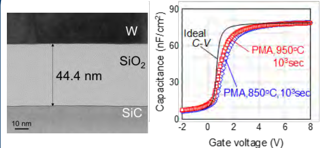
図2 SiCのMOSキャパシタの断面構造と電気特性
