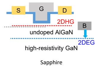
2次元正孔ガス(2DHG)によるGaN系p-チャネルFET
