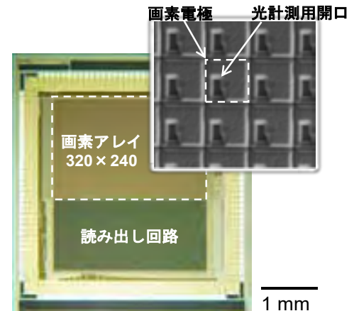
図3. オンチップ光・電位イメージセンサ
