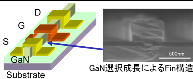
GaNによる立体型トランジスタ: FinFET
