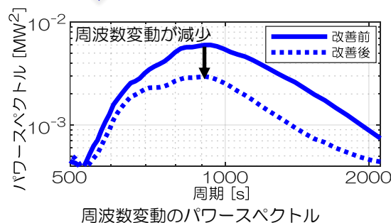
図2 周波数制御システムの最適化による変動のパワースペクトルの改善
