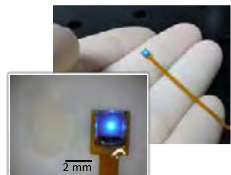
図5. 光遺伝学向け神経光刺激デバイス
