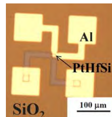
図3 PtHfSiのコンタクト抵抗測定素子
