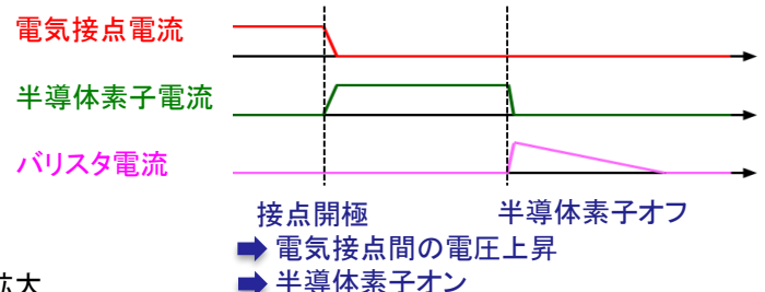
接点電流の半導体素子への転流動作
