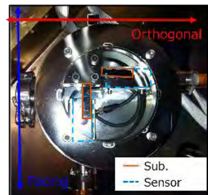
薄膜形成時内部応力の 超高感度観測システム
