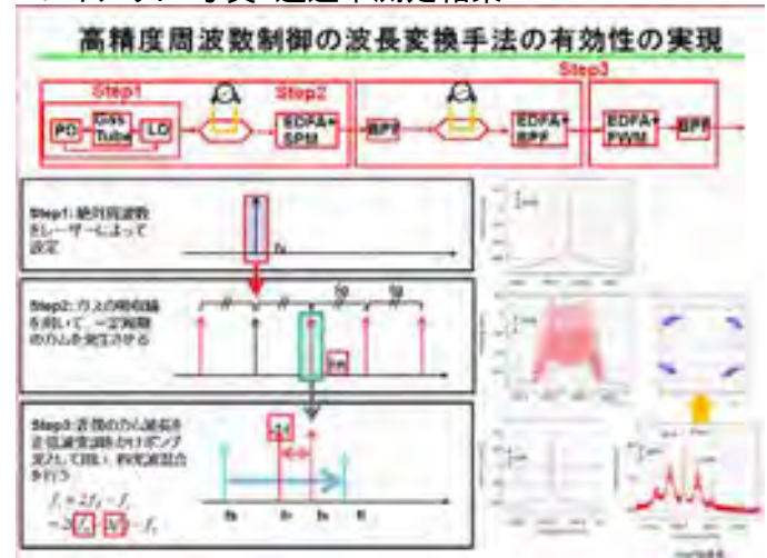
図5 2段コムによるポンプ光を用いた波長デフラグメンテーション技術
