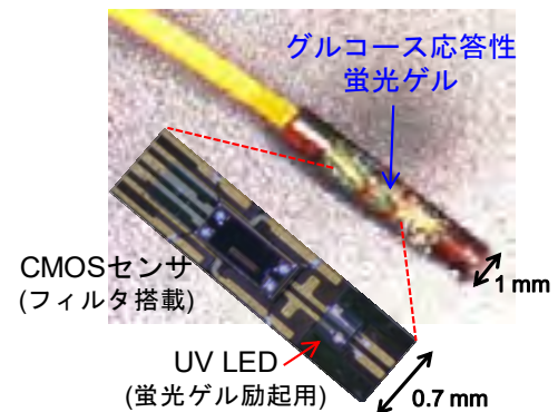
図4. 生体埋め込みグルコースセンサ
