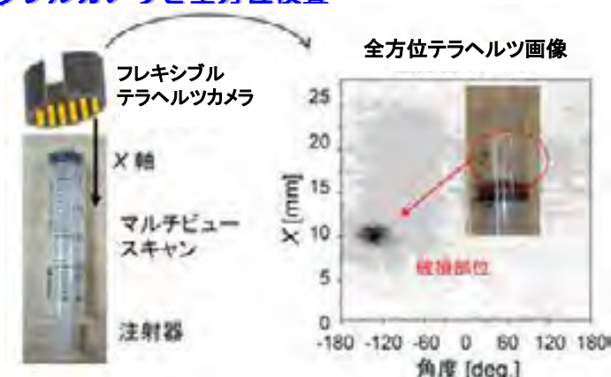
図1 フレキシブルテラヘルツカメラを用いた医療器具(注射器)の360度全方位検査。本撮像デバイスを用いることで、大規模な測定システムなしでの全方位破損検査ができています。
