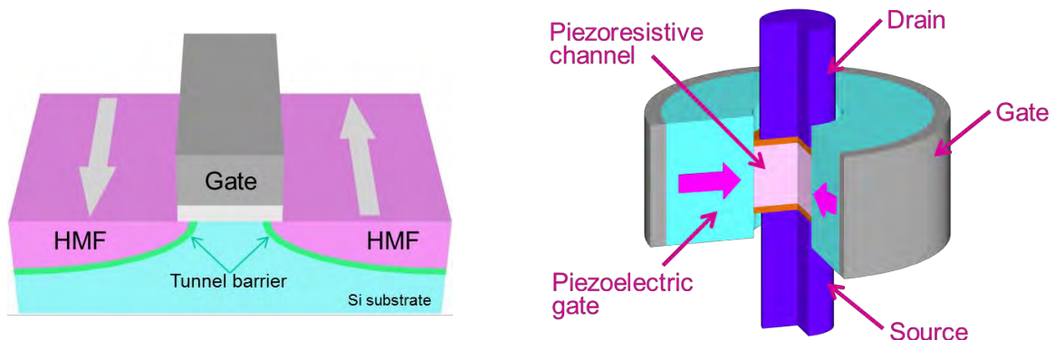
図3 (a) ハーフメタル強磁性体(HMF)ソースドレイン・スピンMOSFET. (b) 圧電エレクトロニック・トランジスタ。
