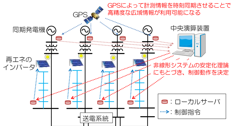
図3 当研究室で提案するスマートインバータによる広域安定化制御システム概念図
