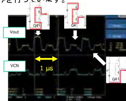
図8 GaN HEMTマルチレベル インバータ集積回路の動作特性
