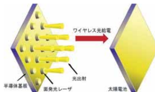
図1 光源と太陽電池による光無線給電
