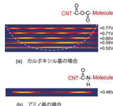
図6: 両端を分子で修飾したカーボンナノチューブ量子ドットの状態密度分布(STS測定による実測結果)
