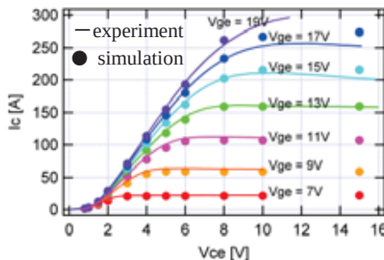
出力特性 (25°C)
