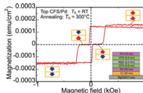
垂直磁化型フルホイスラー合金電極を有したMTJの磁化特性 AIP Advances 8, 055923 (2018).
