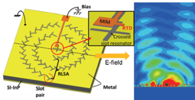
図4 光渦放射RTDテラヘルツ発振器
