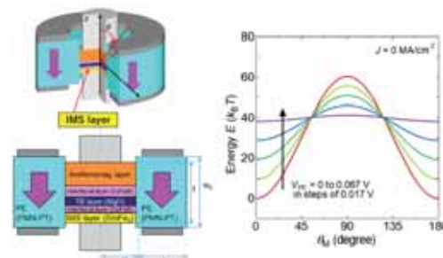
piezoelectronic磁気抵抗変化素子 SSE 128, 194 (2017).
