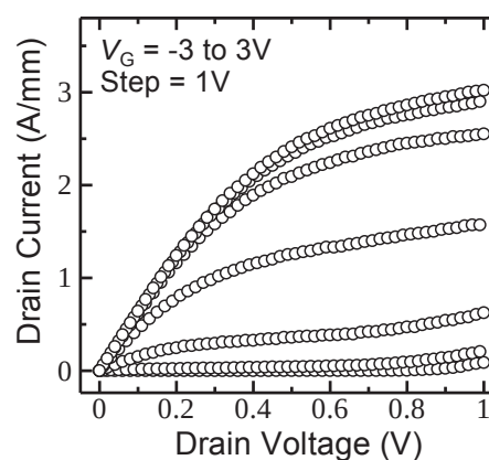
図2 チャネル長50nmの素子のI-V特性
