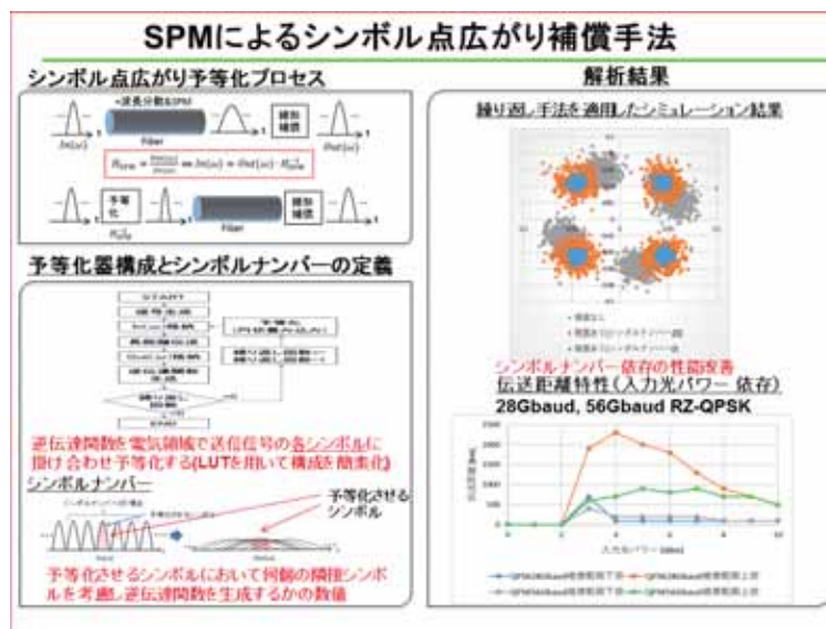
図2 逆伝達関数法を用いた光非線形歪補償技術
