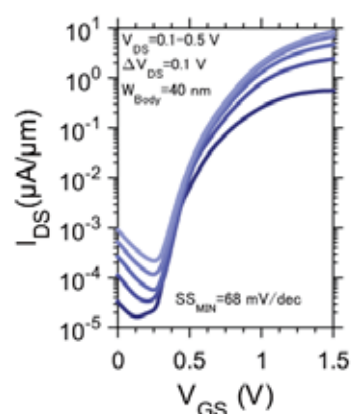
図4 GaAsSb/InGaAsチャンネル縦型トンネルFETのサブスレッショルド特性
