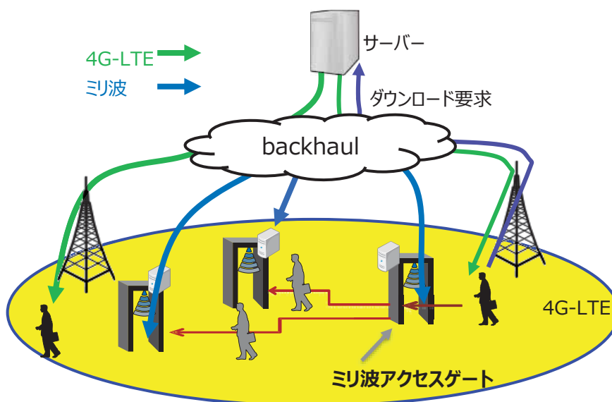
ミリ波超高速アクセスゲートと 4G-LTE を併用した ICN ベースのネットワーク
