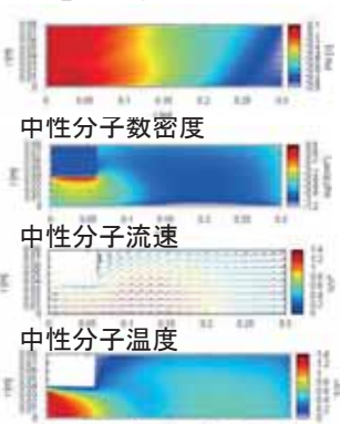
電位分布
