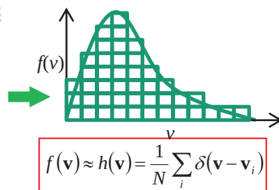
速度分布を統計によって再現
