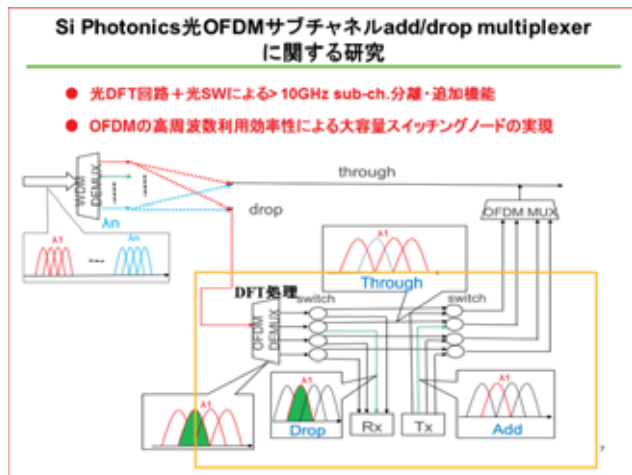
図3 光OFDMサブチャネルadd/drop multiplexer
