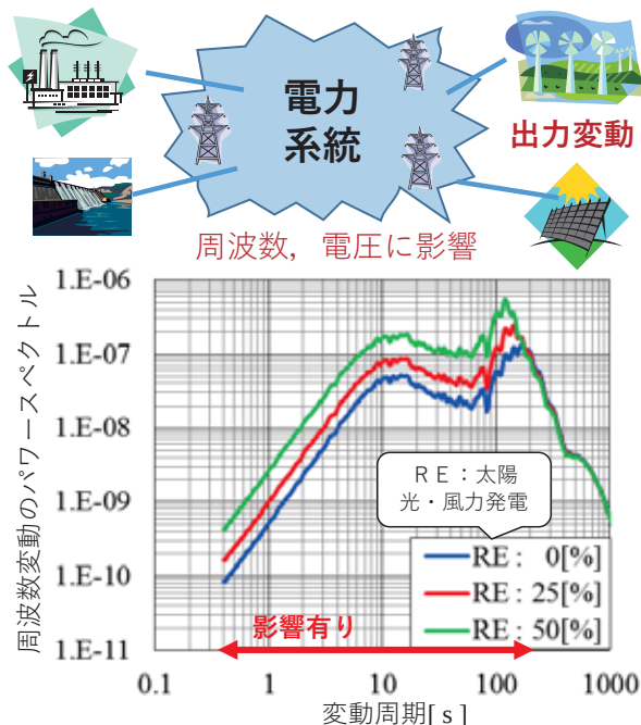
図2 再エネ電源の出力変動が系統周波数に及ぼす影響の評価例
