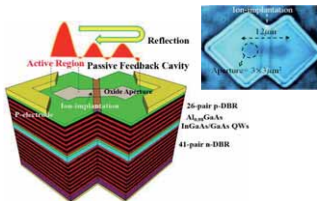
図2 結合共振器面発光レーザ
