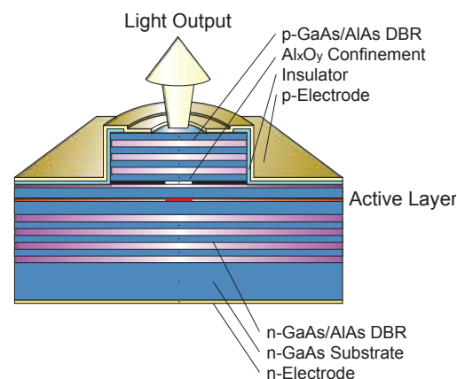
図1 面発光レーザの構造(断面図)。
