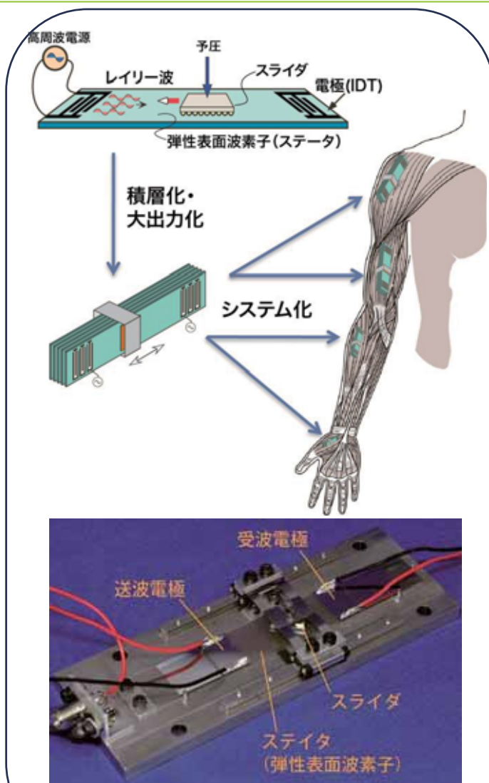
図3. 弾性表面波モータの原理と応用(上) 試作例(下: 最大速度1m/s, 最大推力20N)
