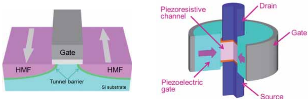
図3 (a) ハーフメタル強磁性体(HMF)ソースドレイン・スピンMOSFET. (b) 圧電エレクトロニク・トランジスタ。
