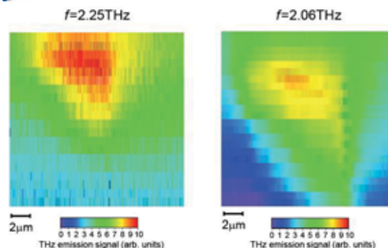
図2 半導体量子素子の電子注入に伴うテラヘルツ発光分布の近接場ナノスケール画像。
