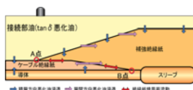
油拡散1/4モデル
