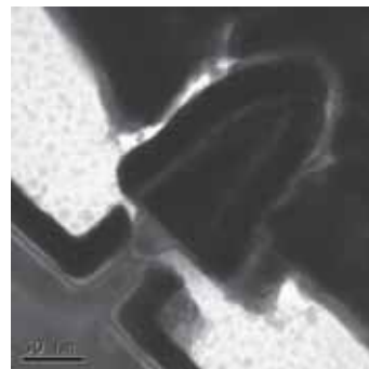
図3 20nm幅のメサを持つ縦型InGaAs TFETの透過電子顕微鏡断面像
