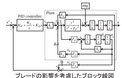
ブレードの影響を考慮したブロック線図
