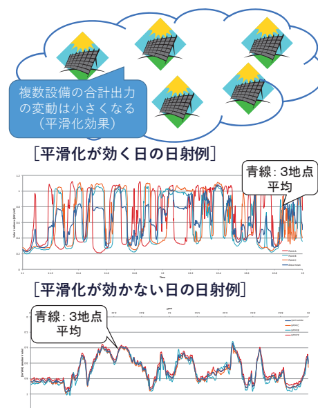
図4 太陽光発電での平滑化効果例
