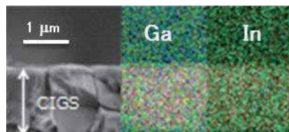
CIGS薄膜の断面電子顕微鏡像とEDSによる組成分布解析
