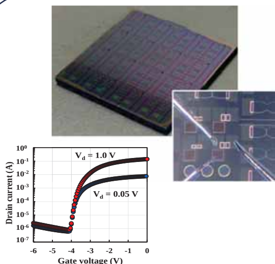
図1 試作したAlGaN/GaN HEMTの写真と特性
