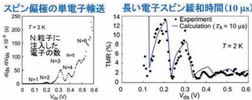
図4. SESTにおける微分電流電圧特性のクーロン階段(左)およびTMRの振動現象(右)の観測。TMR振動の実験を理論でフィッティングした結果、10 \mu sと強磁性金属ナノ微粒子において世界最長のスピン緩和時間を実現した。
