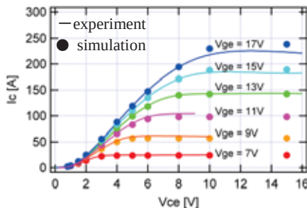
出力特性 (125°C)
