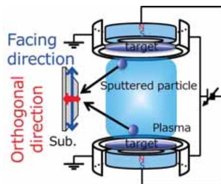
対向ターゲット式スパッタ
