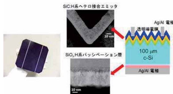
結晶Siヘテロ接合太陽電池
