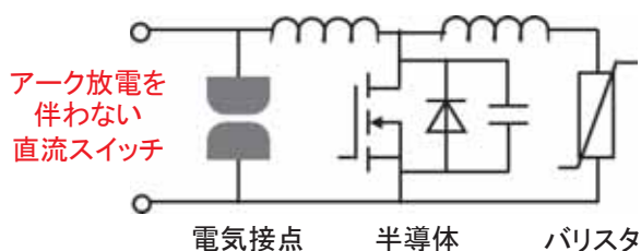
直流ハイブリッド遮断器の構成
