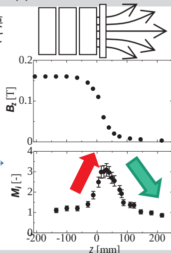
磁気ノズル近傍で測定された磁場強度とイオンマッハ数→
