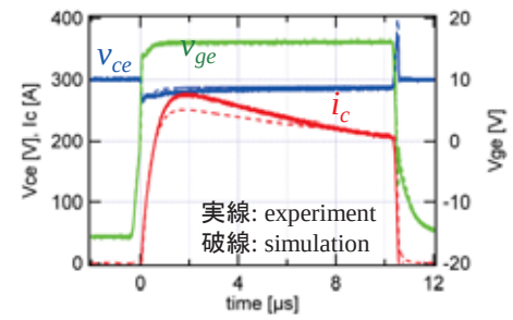
短絡動作波形
