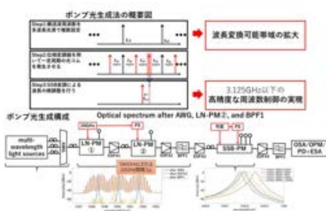
図6 2段コムによるポンプ光を用いた波長デフラグメンテーション技術
