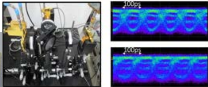
構築したテラヘルツ無線多重通信のシステムと多値伝送時のアイパターン
