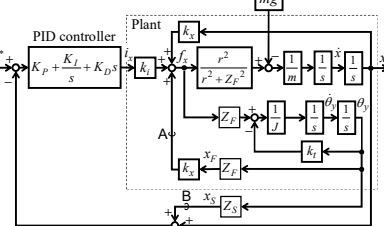
ブレードの影響を考慮したブロック線図
