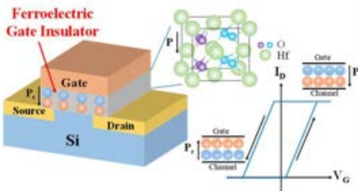
図6 1トランジスタ型Hf系強誘電体メモリ
