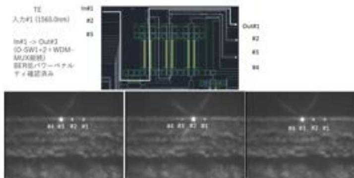
図3 光スイッチング集積素子の出力切り替え動作
