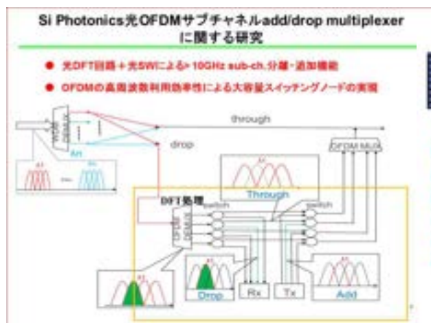
図4 光OFDMサブチャネルadd/drop multiplexer
