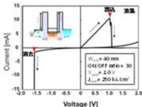
室温でメモリサイクル動作を示す提案素子のI-V特性(実測) (グラフ中左上の図は単体素子のバンドプロフィール)
