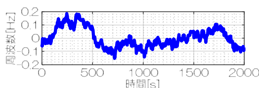
電力システムの周波数シミュレーション結果
