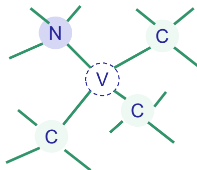
ダイヤモンド中のNVセンター
