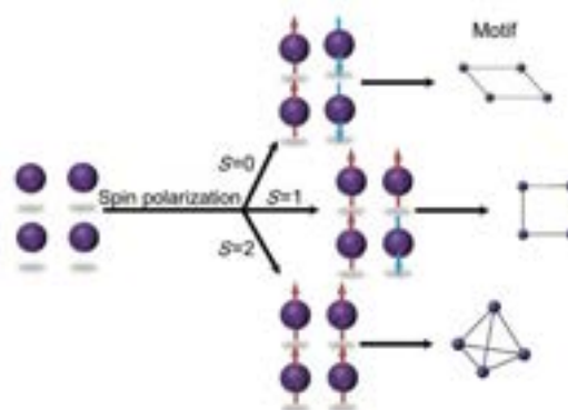
図5 スピンクラスターの形成
