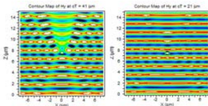
クローキング(透明化)なし 強い散乱があり中央の物質が「見える」
