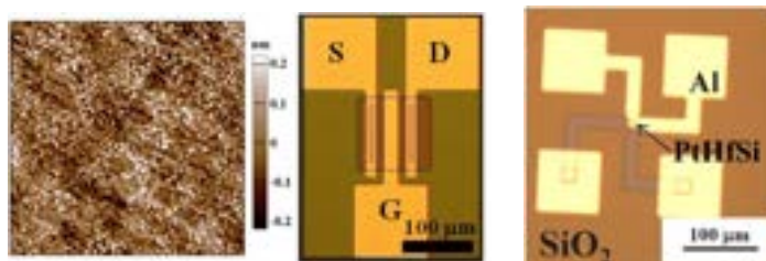
図2 原子レベル平坦Si(100)表面と 図3 PtHfSiのコンタクト抵抗測定素子 Hf系MONOSデバイス
