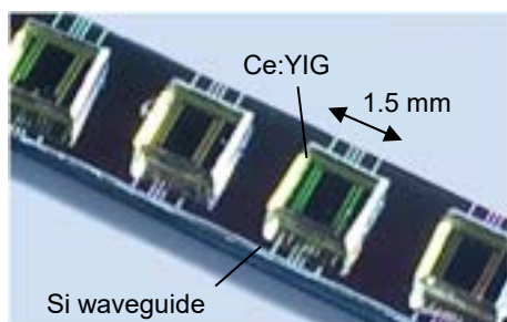
Si導波路光アイソレータ
