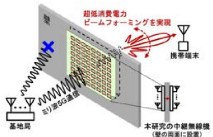
図4. 電源不要の無線電力伝送型ミリ波5G無線中継機
