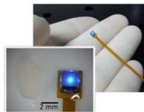
図5. 光遺伝学向け神経光刺激デバイス
