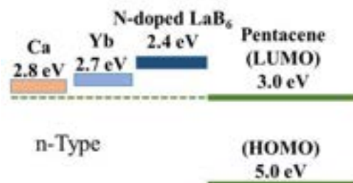
図5 ペンタセンと低仕事関数金属のバンド構造
