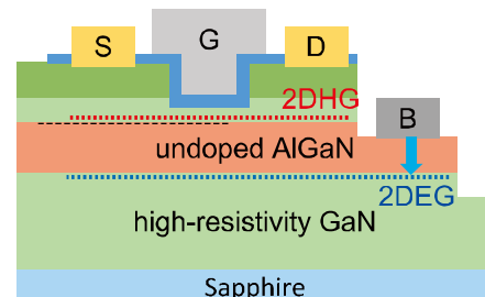
2次元正孔ガス(2DHG)によるGaN系p-チャンネルFET
