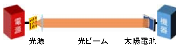
図1 ビーム光源と太陽電池による光無線給電
