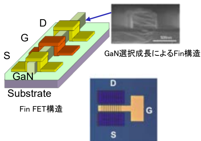
Finチャネル10本並列のトランジスタ製作例
