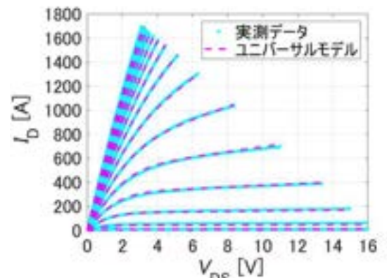
図2 実測値とモデルの V_{DS} と I_D の関係
