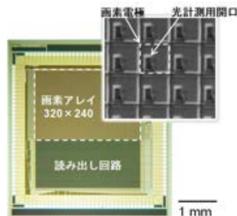
図3. オンチップ光・電位イメージセンサ
