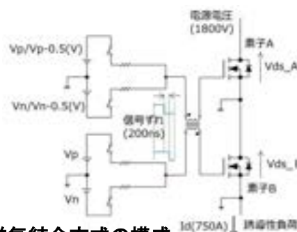
図3 磁気結合方式の構成
