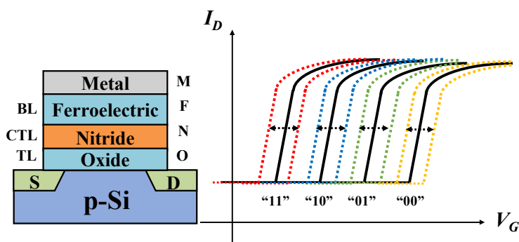
図1 FeNOS型不揮発性メモリと動作特性
