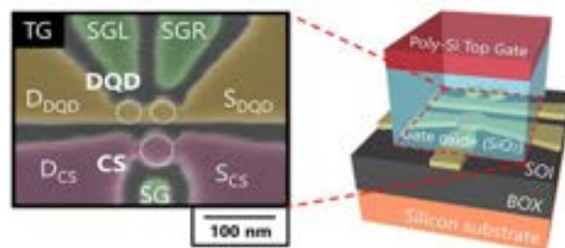
MOS構造を利用したシリコン量子ドットデバイス
