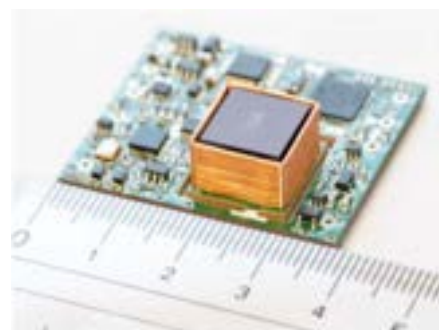
図7. 超低消費電力な小型原子時計
