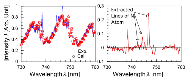
N_2 1PSに埋もれたN原子発光線抽出
