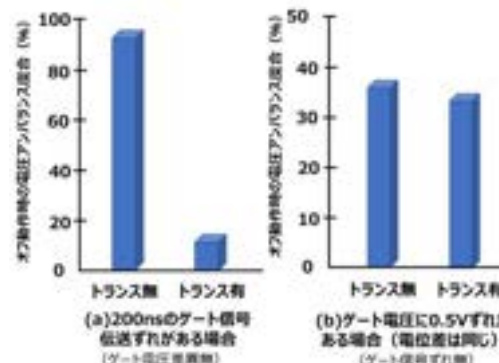
図4 磁気結合トランス有無とオフ動作時の電圧アンバランス度合の関係
