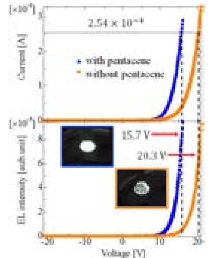
図2. 透明電極上にペンタセンを挿入した有機ELデバイスの特性
