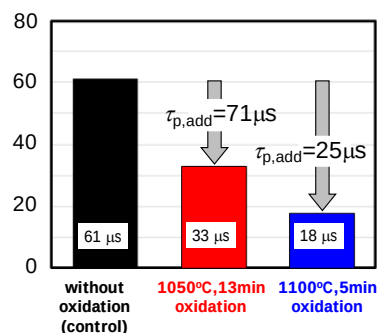
図1 少数キャリア寿命の高精度抽出
