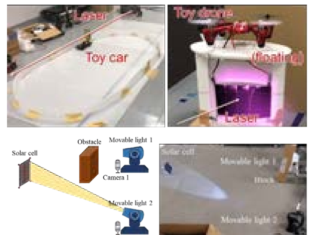
図4 事例紹介: 玩具の自動車(左上)・ドローン(右上)への給電や、複数光源による高機能給電(下)
