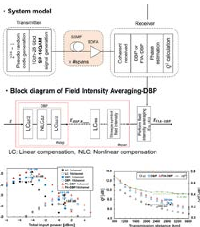
図2 強度平均化法を用いた光非線形歪補償技術
