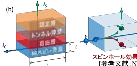
図2. 第2世代のSTT-MRAMと第3世代のSOT-MRAMの比較
