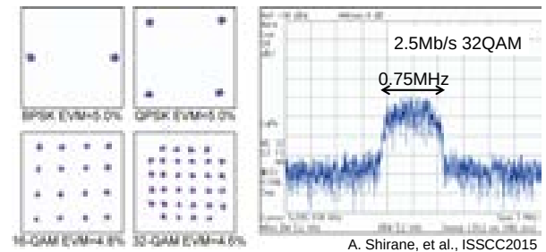
図2. 直交ボックスキャタリング回路技術
