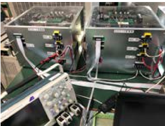
直流遮断器評価装置の外観
