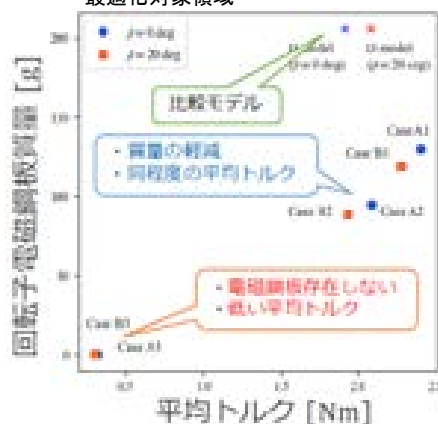
最適化結果(平均トルク対重さ)
