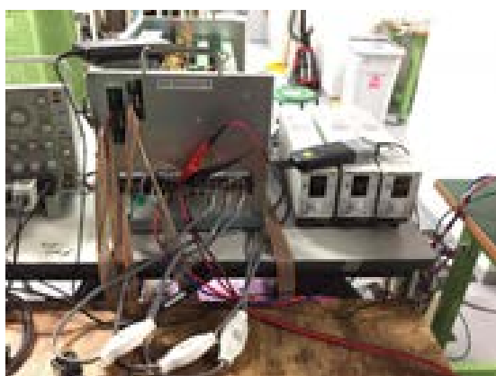
インダクタの小型・軽量化が実現可能な 補助変換器を用いた双方向チョップパの外観図
