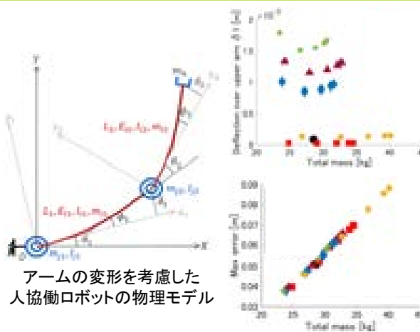
材料別のアームの変形と手先誤差
