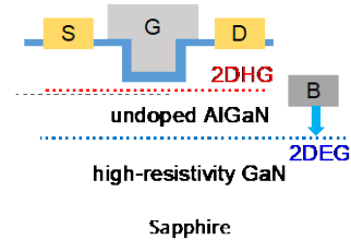
2次元正孔ガス(2DHG)によるGaN系p-チャネルFET
