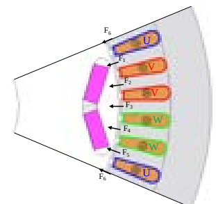
零相電流を用いたラジアル力低減
