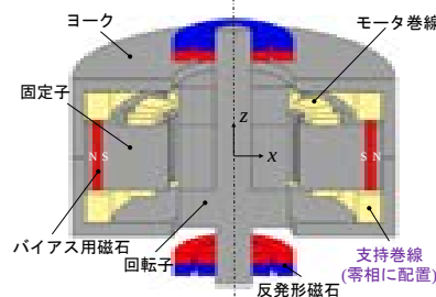
1軸制御ベアリングレスモータ(零相電流で磁気支持)
