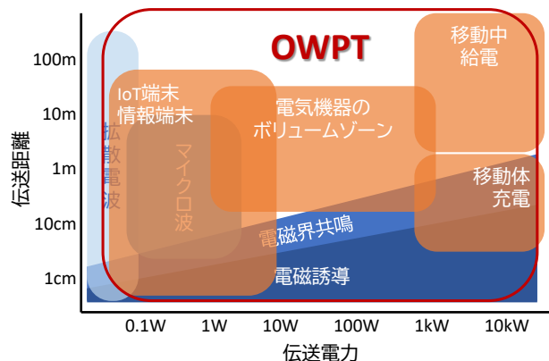
図2 光無線給電は小型軽量・長距離・大電力のため, 様々な機器・場面への利用が期待される。
