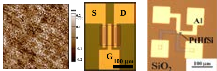
図2 原子レベル平坦Si(100)表面と 図3 PtHfSiのコンタクト抵抗測定素子
