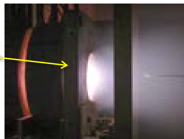
磁気ノズルから噴出される超音速膨張アークジェット
