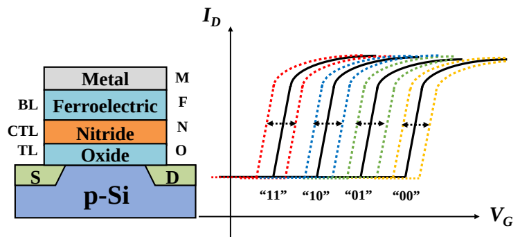
図1 FeNOS型不揮発性メモリと動作特性
