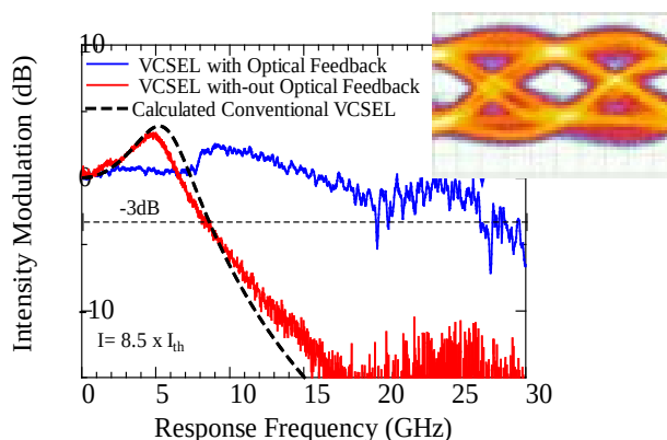
図3 結合共振器面発光レーザの高速変調
