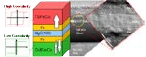
垂直磁化p-MTJの構造図と断面TEM像 JAP 103, 07A911 (2008).
