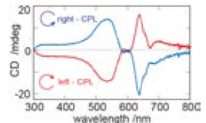
図3. キラルPDAのCDスペクトル
