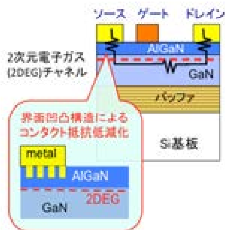
HEMT構造と新コンタクト形成技術
