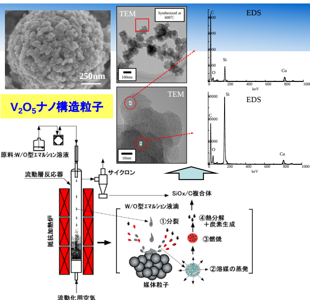
高温流動層を用いた \text{SiO}_x/\text{C} 微粒子合成プロセス
