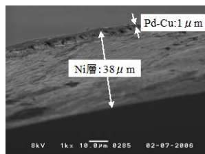
図3 逆ビルドアップ法を用いた金属複合水素透過膜
