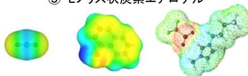
④ 量子化学計算で得られる分子情報
