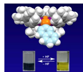
HFセンシング (左) とミュオニウム付加体を示すスペクトル (右)
