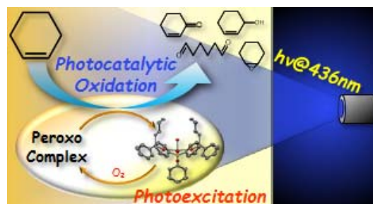
可視光応答型酸素化触媒としてのウラン錯体機能開拓
