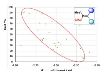
ホスファアルケン-金錯体の触媒活性と配位子のLUMO準位の相関を示すグラフ (左) と新規P2配位子 (右)
