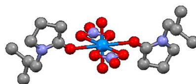
(左) 模擬FP元素およびU(VI)を含む3 M硝酸溶液にNRP (R = iso-propyl)を加えた際の選択的U(VI)沈殿生成の様子。 (右) 沈殿中に含まれるウラン(VI)錯体の分子構造。
