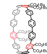
[7]ヘリセン
