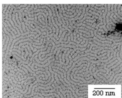
有機-シリカナノ複合体の電子顕微鏡写真
