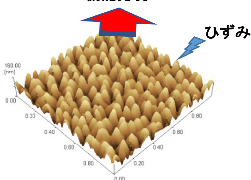
垂直配向薄膜(AFM画像)
