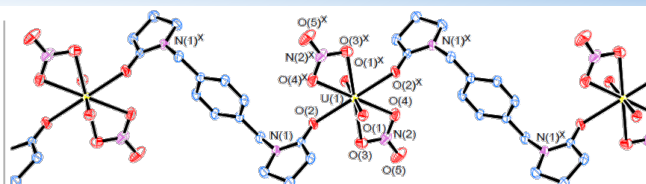
架橋ピロリドン誘導体を含む硝酸ウラニル1次元鎖配位高分子 【NUMAP法による使用済み核燃料簡易再処理技術開発】
