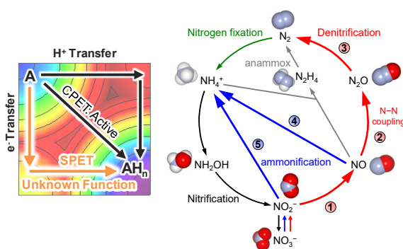
図2 電子-プロトン輸送の制御に基づく窒素代謝の人工的再現
