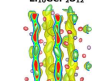
LGPS系材料のLi + 伝導パス
