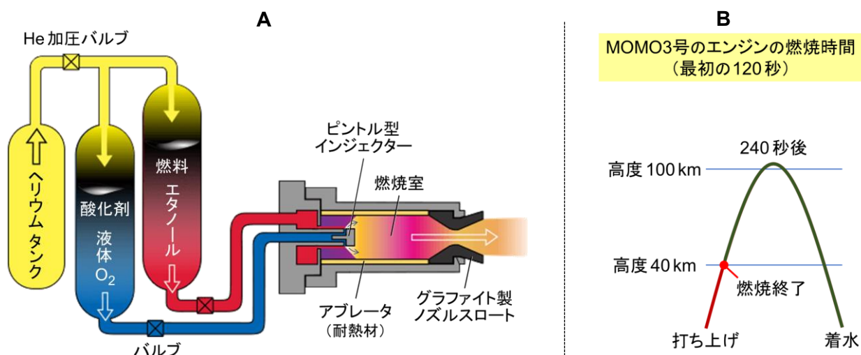
図 2. 観測ロケット MOMO のエンジンの仕組み(A)と MOMO3 号機の航跡(B)。エンジンによる動力飛行は最初の約 120 秒間で、あとは慣性飛行で高度 113 km に達した。
